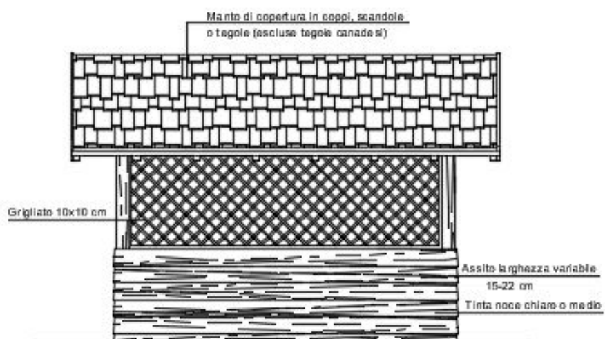
VISTA LATERALE
